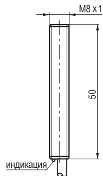
Габаритный чертеж
